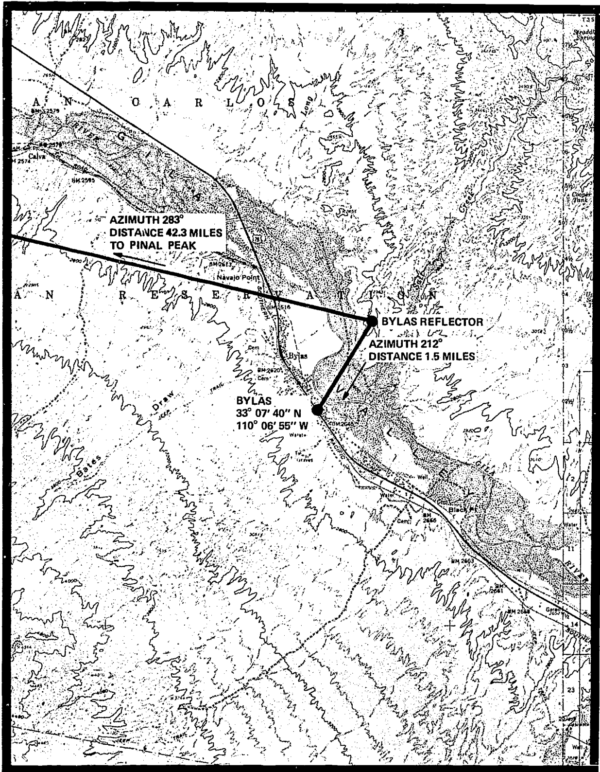
Figure B.4. Bylas and Bylas Reflector Site Map.
